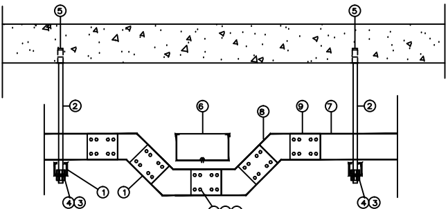
DETALHE GNERICO DE CRUZAMENTO DE ELETROCALHAS SEM ESCALA
